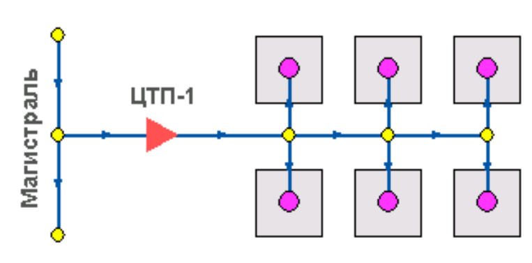
Рисунок 5 - Изображение ЦТП
